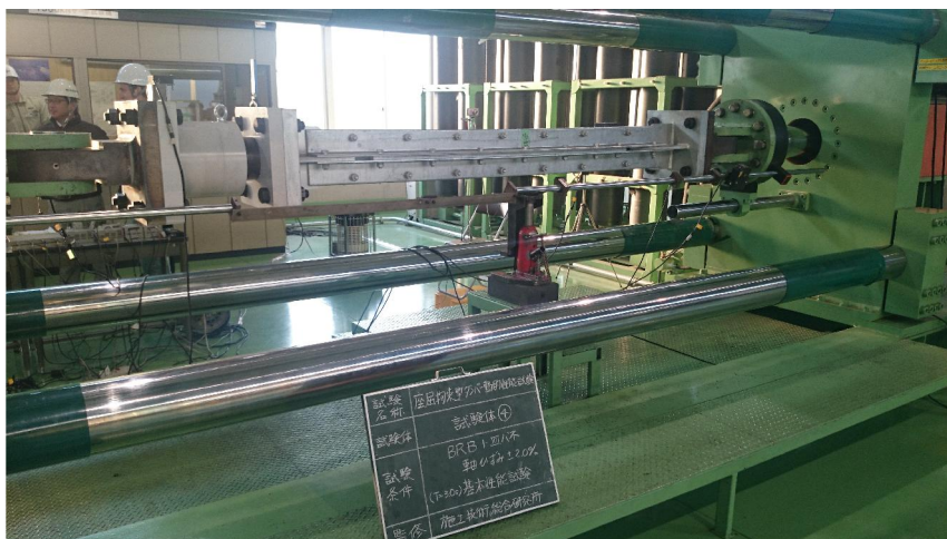
座屈拘束型ダンパー 試験体
